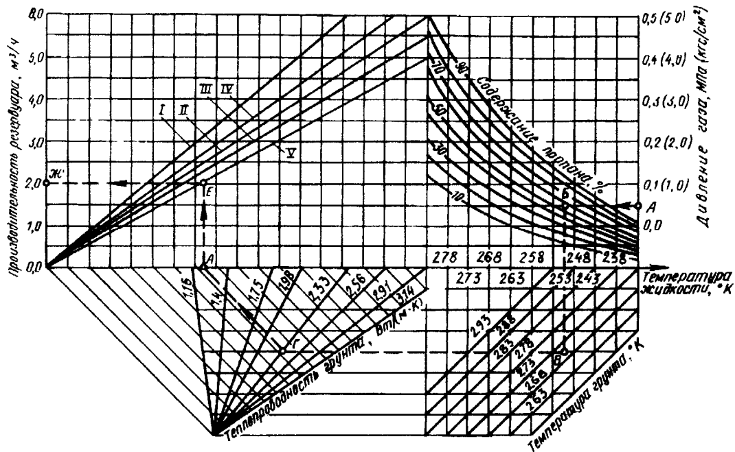
Номограмма для определения производительности резервуара сжиженного газа вместимостью 2,5 и 5 m^3 (подземного)
